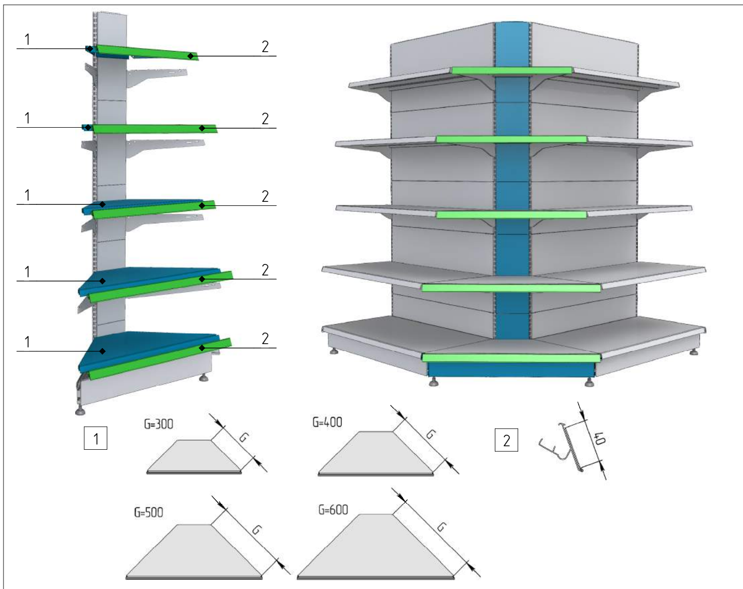
1 Полка угловая
