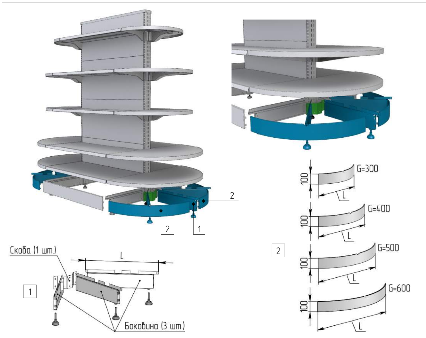
1 Комплект боковин в сборе со скобой
